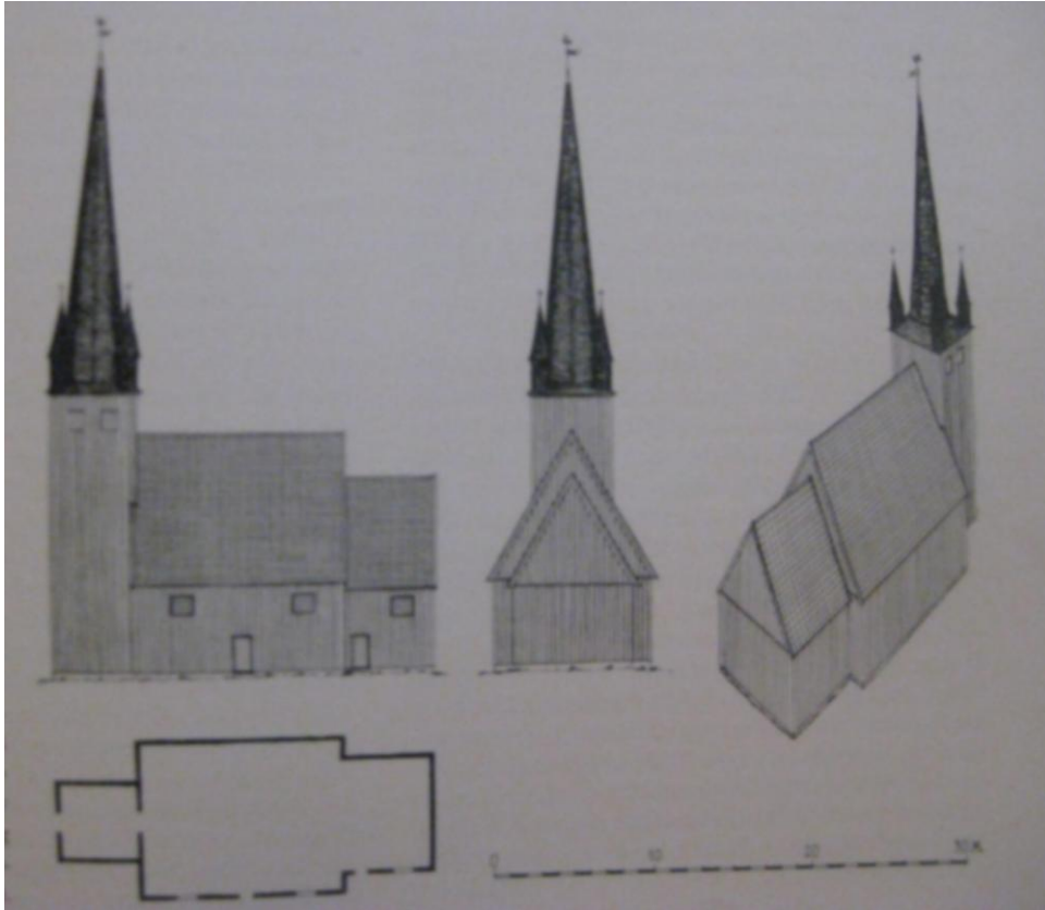
Rekonstruksjonstegning av Fet kirke slik Jens Nilssøn kan ha sett den.
